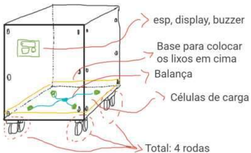
IMAGEM 3: Desenho a mão livre com projeto de Caixa de coleta ciberfísica.
