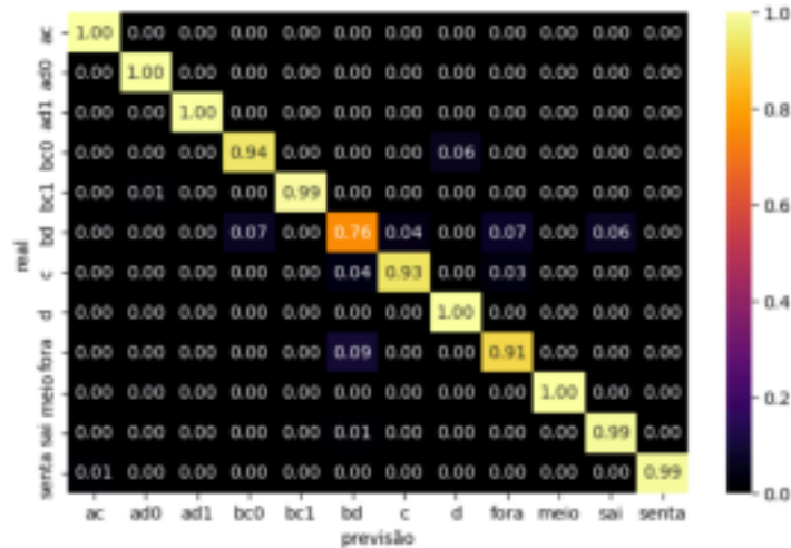
Figura 3 - Matriz de confusão.
